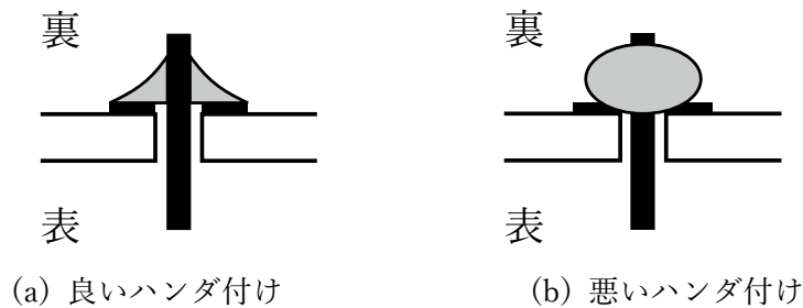
図1 良いハンダ付けと悪いハンダ付け
