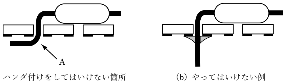
図2 ハンダ付けをする場所
